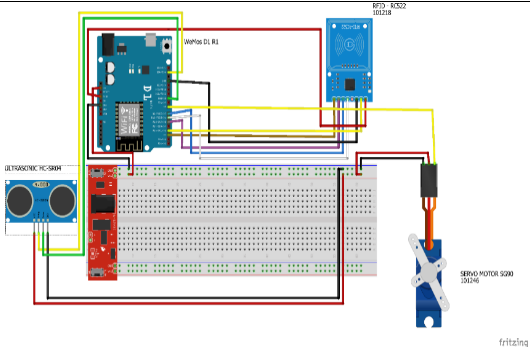
Gambar 1. Rangkaian Pintu Portal Otomatis
