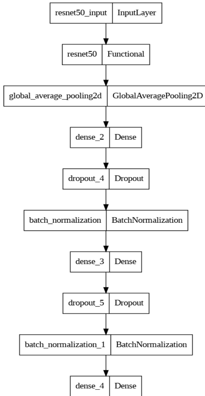
Gambar 15 Rancangan Model Arsitektur ResNet-50
