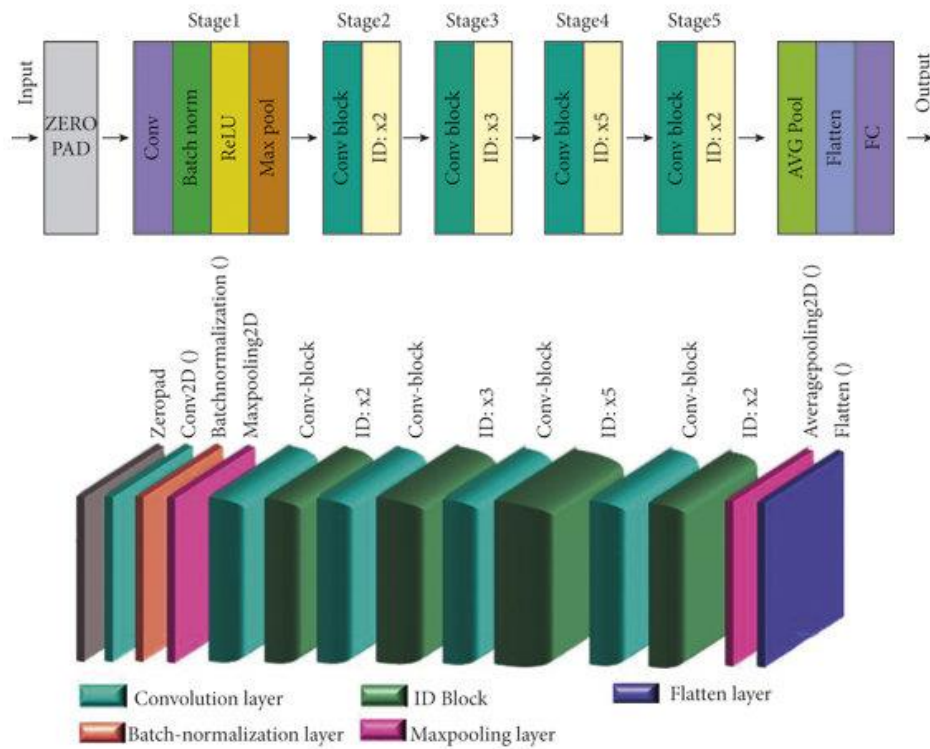
Gambar 14 Visualisasi Resnet-50
