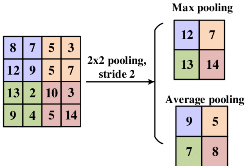
Gambar 12 Pooling Layer
