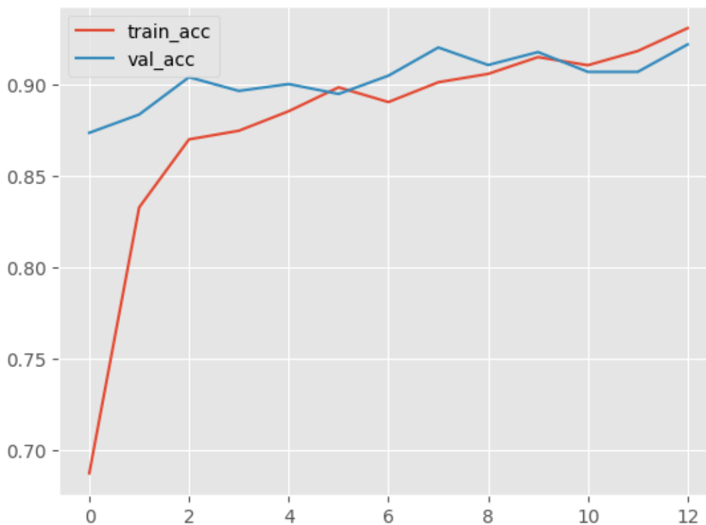
Gambar 17 Train dan Validation Accuracy pada Model ResNet-50
