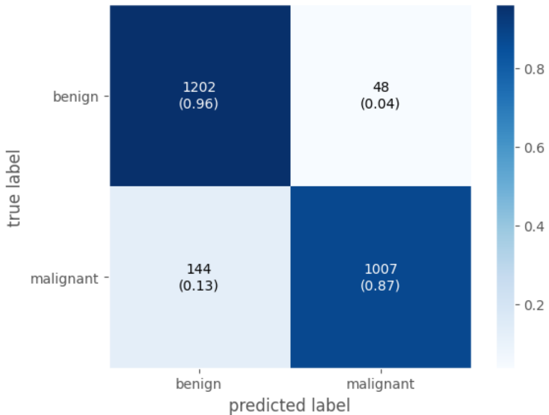
Gambar 18 Confusion Matrix pada Model ResNet-50
