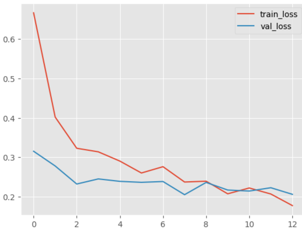
Gambar 16 Train dan Validation Loss pada Model ResNet-50
